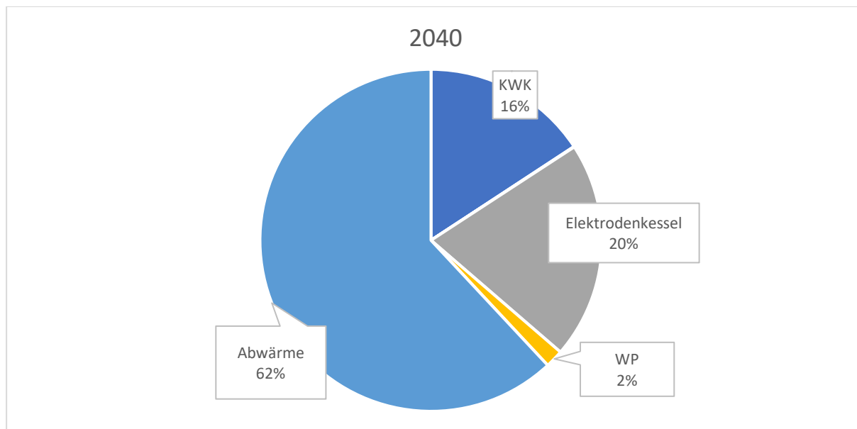
Abbildung 28: Nahezu klimaneutrale Fernwärmeversorgung Rudolstadt-Schwarza 2040 durch TWS gemäß vorliegender Transformationsplanung
