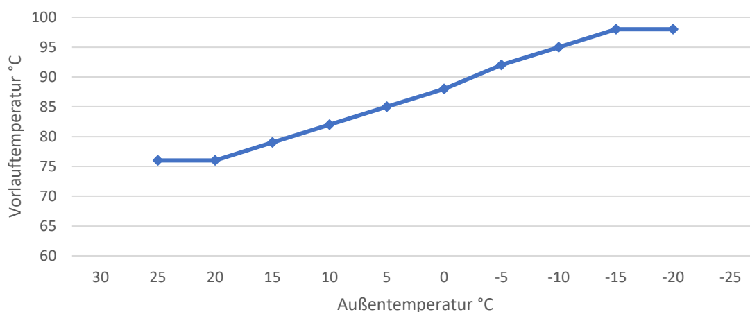
Abbildung 26: Temperaturfahrkurve für das Heißwassernetz Rudolstadt-Schwarza
